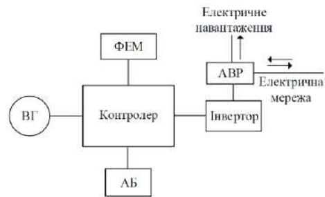
Рис.3 - Структурна схема роботи фотоелектричних модулів та вітрогенератора
