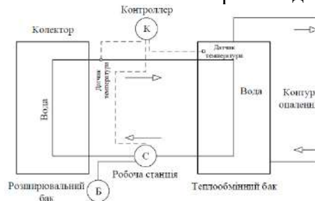
Рис.2 - Структурна схема роботи сонячного колектора
